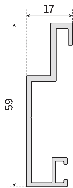
MKL4427 531 kg/m
