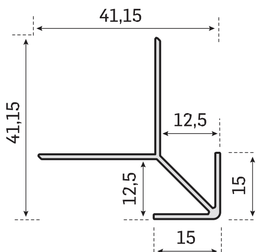
MKL4410 - 0,298 kg/mt
