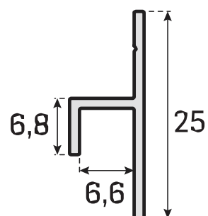
MKL4421 - 0,125 kg/mt
