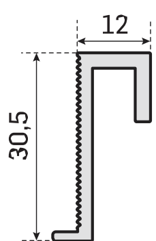
MKL4423 - 0,268 kg/mt
