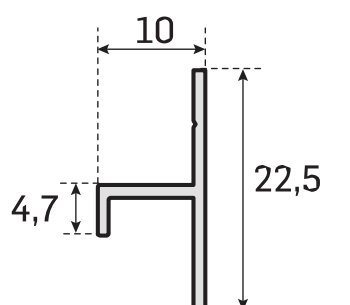
MKL4419 - 0,106 kg/mt Yatay Derz
