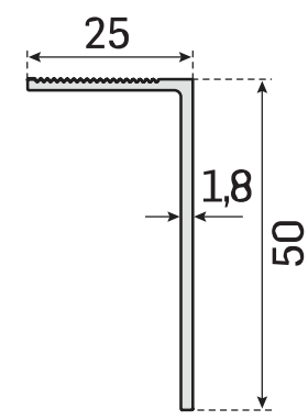
MKL4403 0,347 kg/mt
