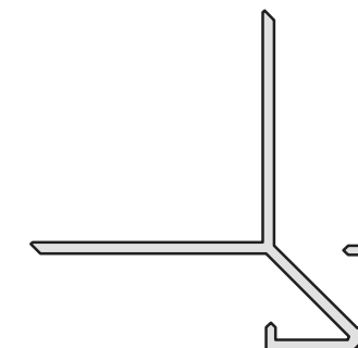
MKL4409 - 0,279 kg/m
