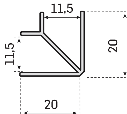
MKL4411 - 0,200 kg/mt
