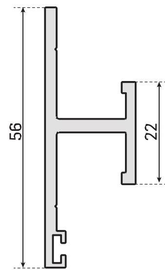
MKL4426 - 0,634 kg/mt
