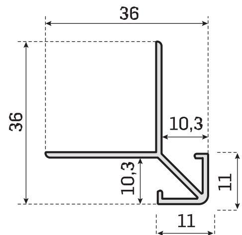
MKL4409 - 0,279 kg/mt
