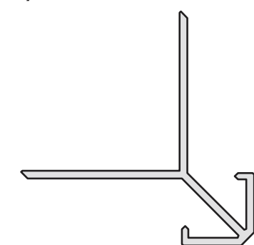
MKL4409 0,279 kg/m
