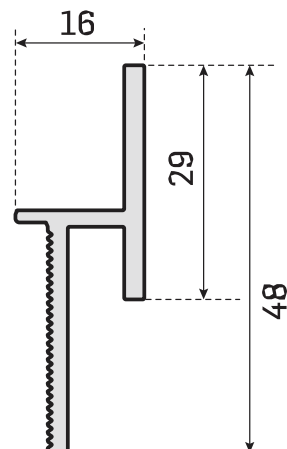
MKL4425 - 0,379 kg/mt
