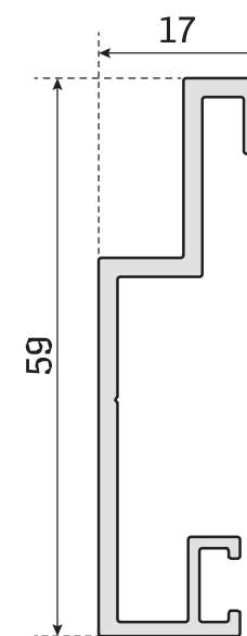
MKL4427 - 0,531 kg/m
