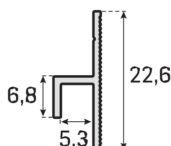
MKL4422 - 0,106 kg/mt
