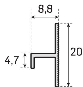
MKL4420 - 0,089 kg/mt Düşey Derz
