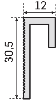
MKL4424 - 0,255 kg/mt
